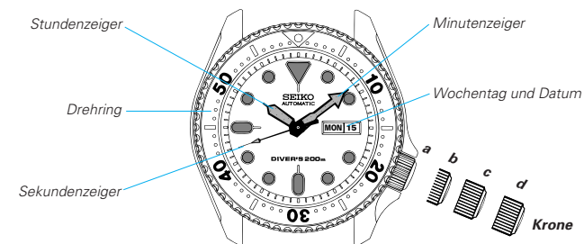
a: Einschraubposition b: Normalposition c: 1. Einrastposition d: 2. Einrastposition
